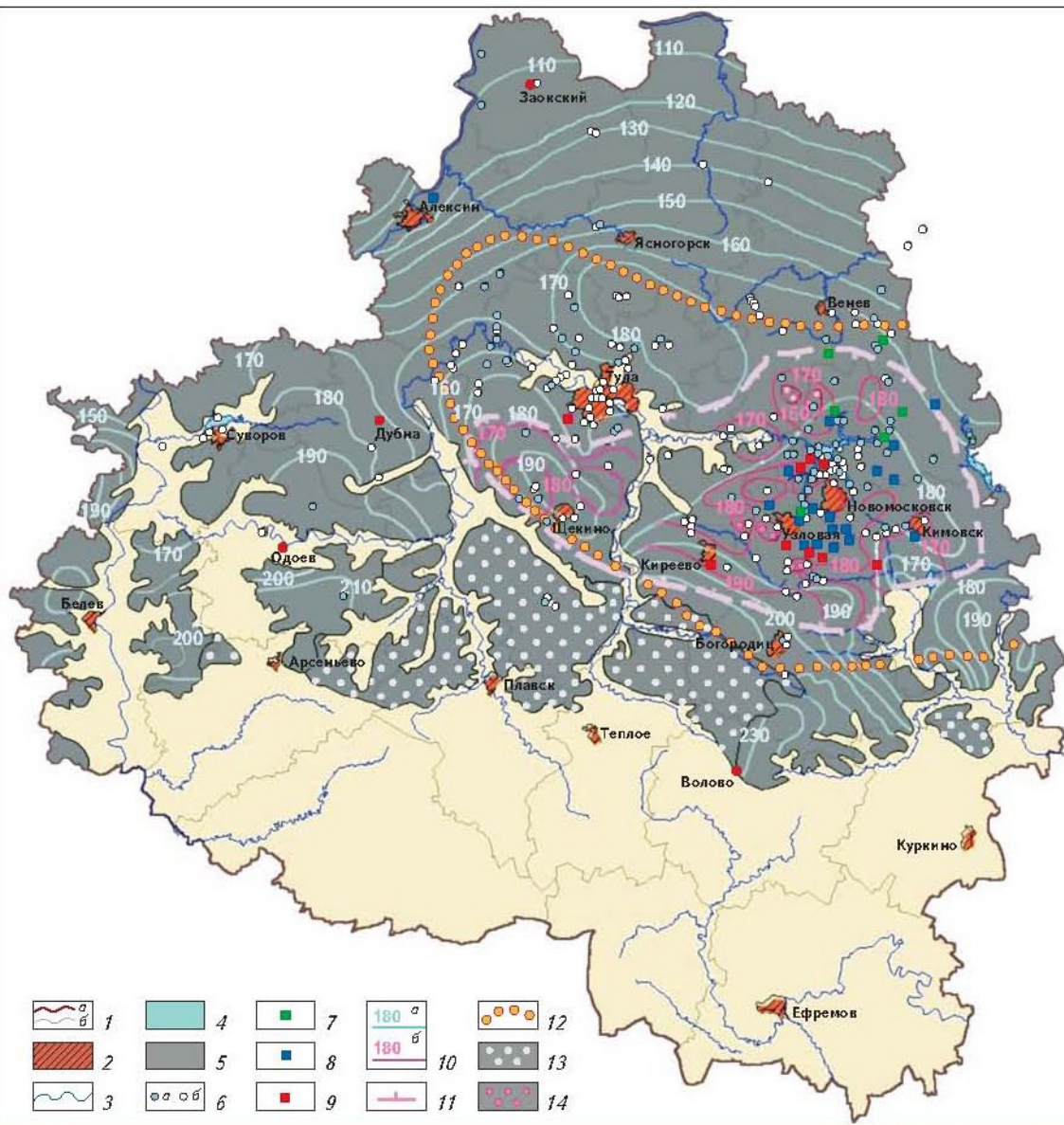
Рис. 1.30. Схематическая карта состояния яснополянского водоносного горизонта (Тульская область) (Тульский ТЦ ГМСН, ФГУП “Геоцентр-Москва”)
