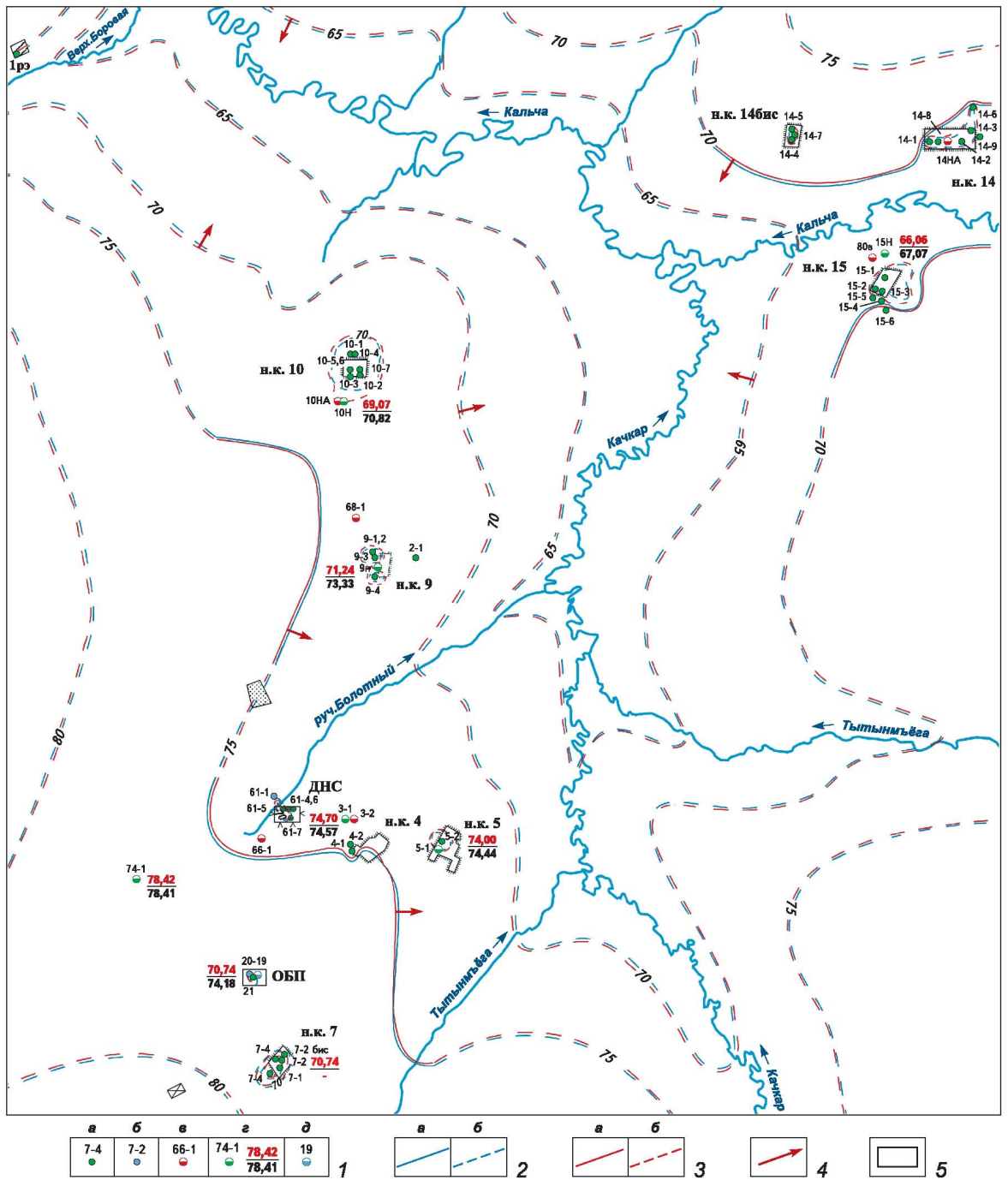
Рис. 1.48. Схематическая карта гидроизоэпез новомихайловского водоносного горизонта в пределах Кальчинского месторождения нефти (ГУП ТО ТЦ “Тюменьгеомониторинг”)
