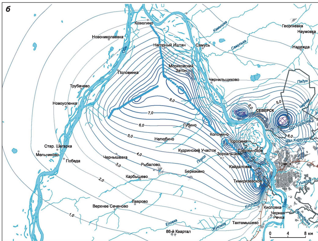
Рис. 1.29. Изменение среднегодовых значений снижения уровней подземных вод в пределах Обь-Томского междуречья за весь период работы водозабора (ОАО "Томскгеомониторинг")
