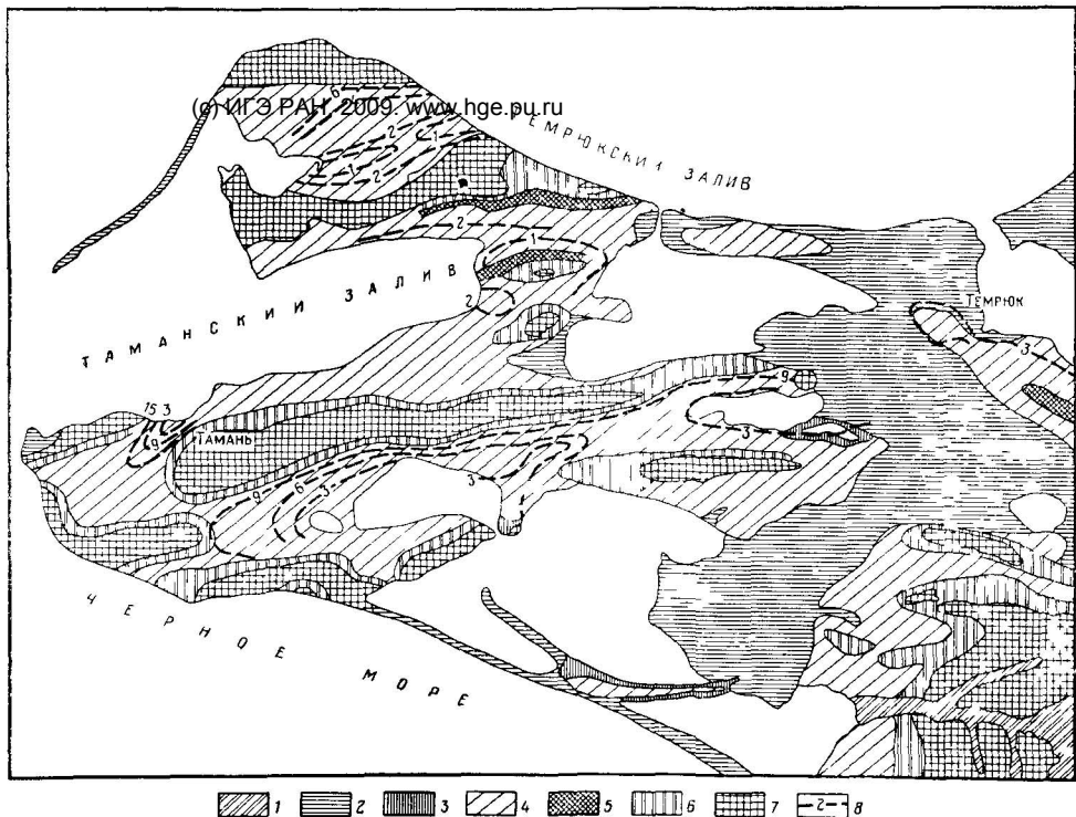
Рис 36 Схематическая карта подземных вод четвертичных и дочетвертичных отложений Таманского гидрогеологического района (Составил В А Лободин)
