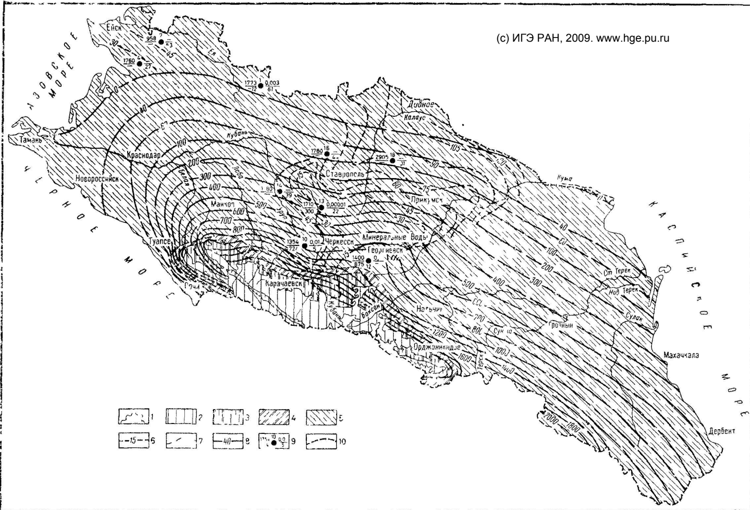
Рис. 24 Схематическая карта пьезоизогипс и химического состава вод отложенный докембрия — палеозоя (Составили Г. М. Сухарев, Ю. К. Тарануха, Н. С. Погорельский)
