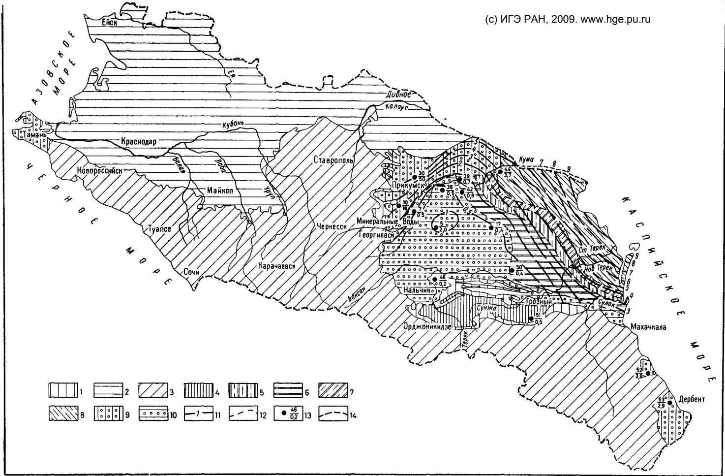
Рис. 10. Схематическая гидрохимическая карта водоносного комплекса отложений ачкагыльского яруса (Составил Н. С. Погорельский)
