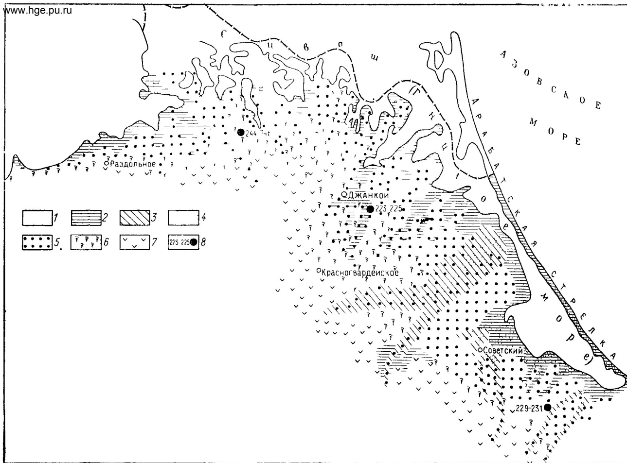
Рис. 24 Схематическая карта элементов баланса грунтовых вод северо-восточной части Равнинного Крыма в естественных условиях Составила Е. А. Ришес
