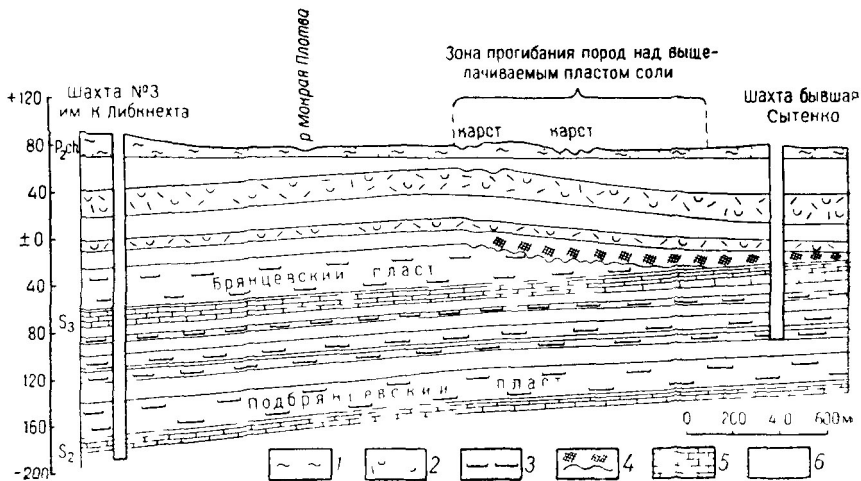
Рис 115 Геологический разрез по линии шахты № 3 им. К. Либкнехта — шахта б. Сытенко (по Л. Н. Нестеренко)
