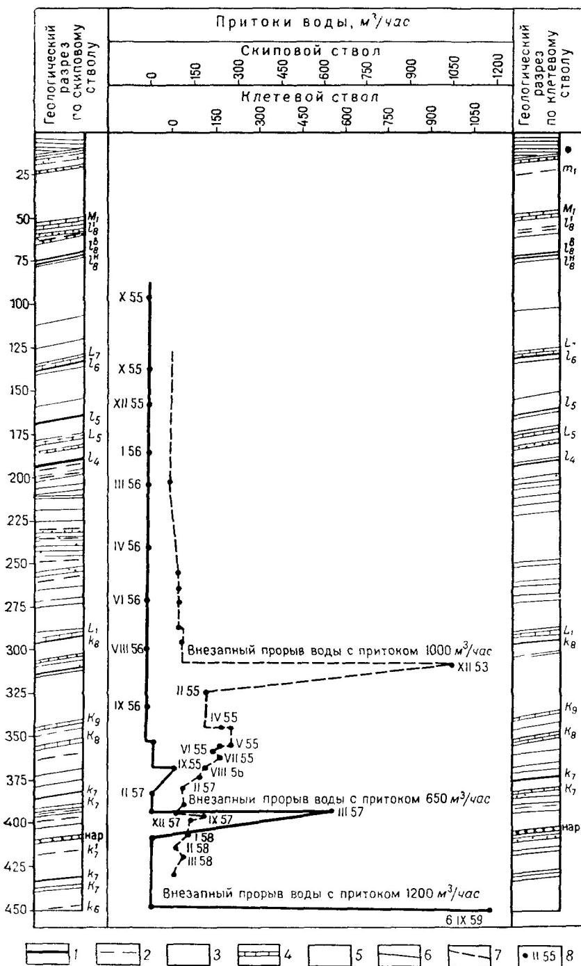
Рис 93 Притоки воды в стволы шахты «Центральная Первомайская» 1 — угли рабочей мощности 2 — угли нерабочей мощности 3 — песчаники 4 — известняк 5 — аргиллиты и алевролиты 6 — приток по скиповому стволу 7 — приток по клетевому стволу 8 — дата определения притока
