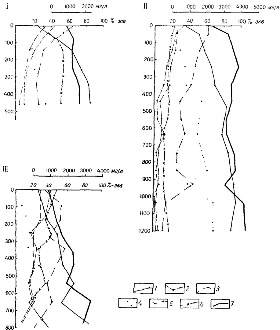
Рис 73 Изменение с глубиной минерализации и содержания основных ионов в подземных водах
