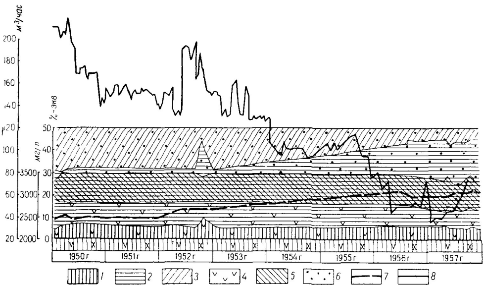
Рис. 71. Изменение химического состава вод в шахте «Ново-Гродовка»
