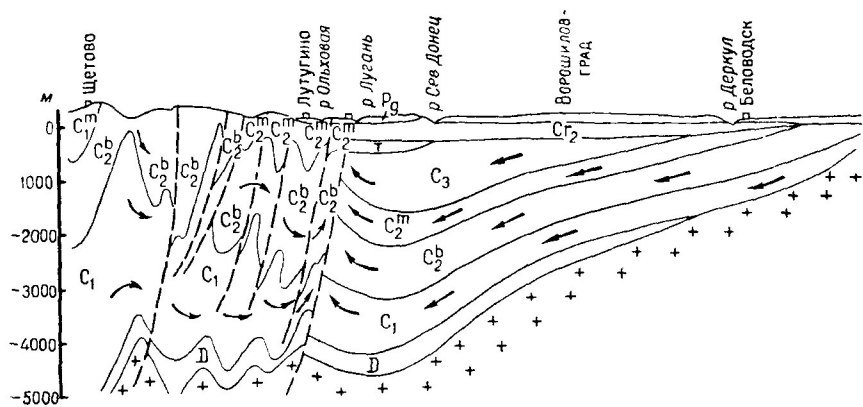
Рис 66 Схема движения и разгрузки подземных вод в зоне северных региональных разломов
