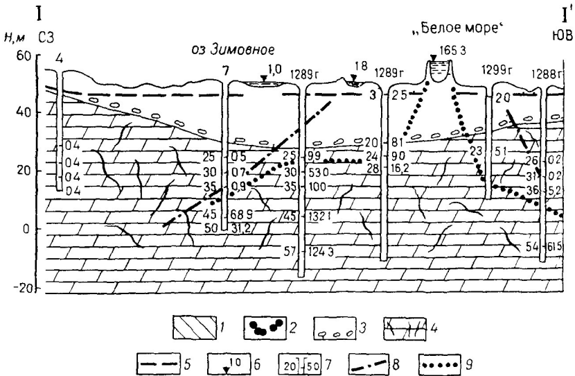
Рис 63 Изменение состава подземных вод в районе «Белого моря» з-да «Донсода» (по А Н Власовскому)
