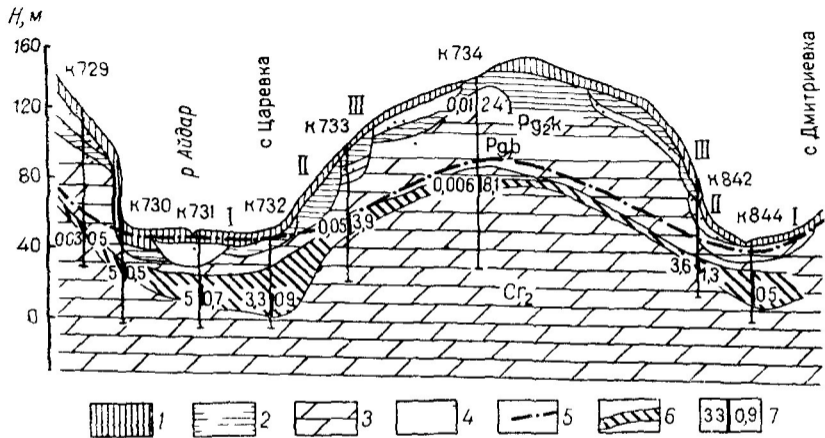
Рис. 61. Гидрогеологический разрез по линии сел Царевка — Дмитриевка (Старобельский район Ворошиловградской области)
