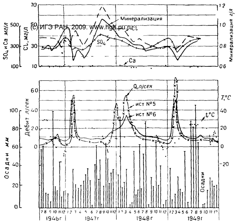
Рис 51 Изменение дебита, химического состава и температуры воды в источниках на площади открытого карбона
