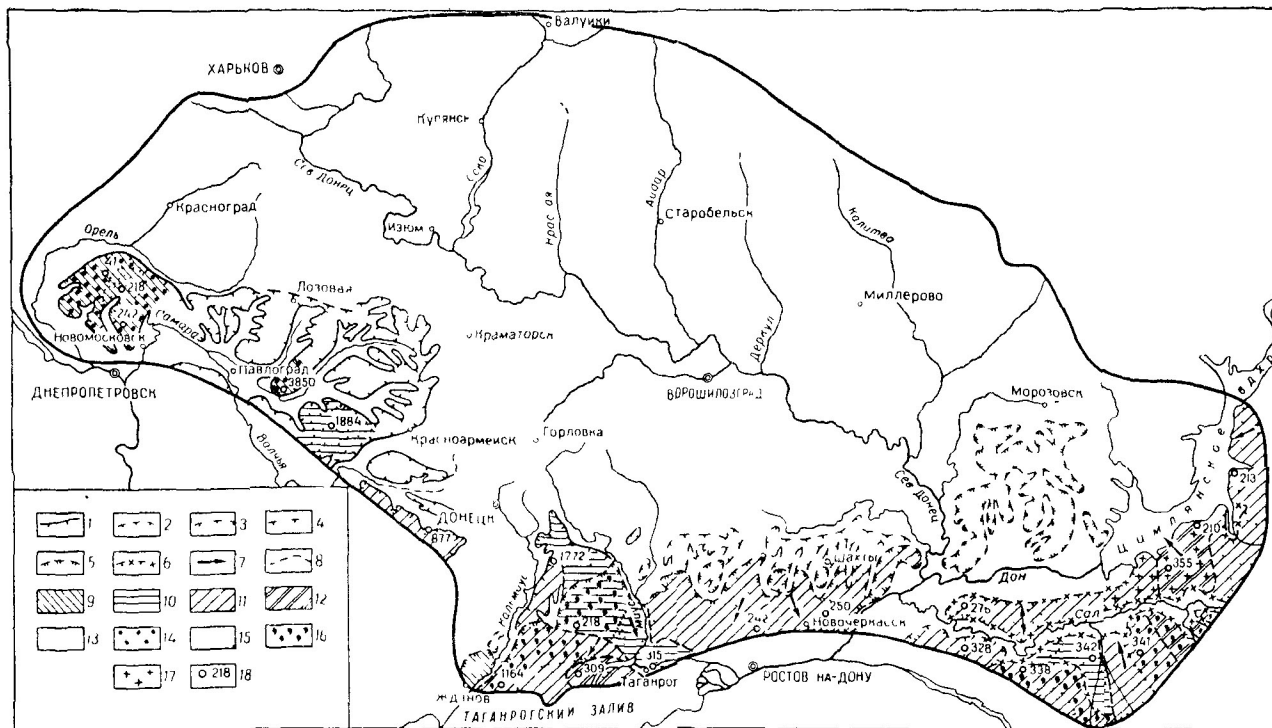
Рис. 47. Схематическая карта распространения водоносных горизонтов в сарматских, понтических, верхнелиоценовых и ергенинских отложениях. (Составил В. Г. Василенко)
