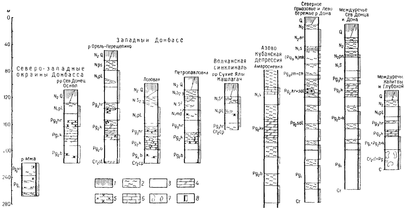
Рис 44 Сопоставление водоносных горизонтов палеогеновых и неогеновых отложений
