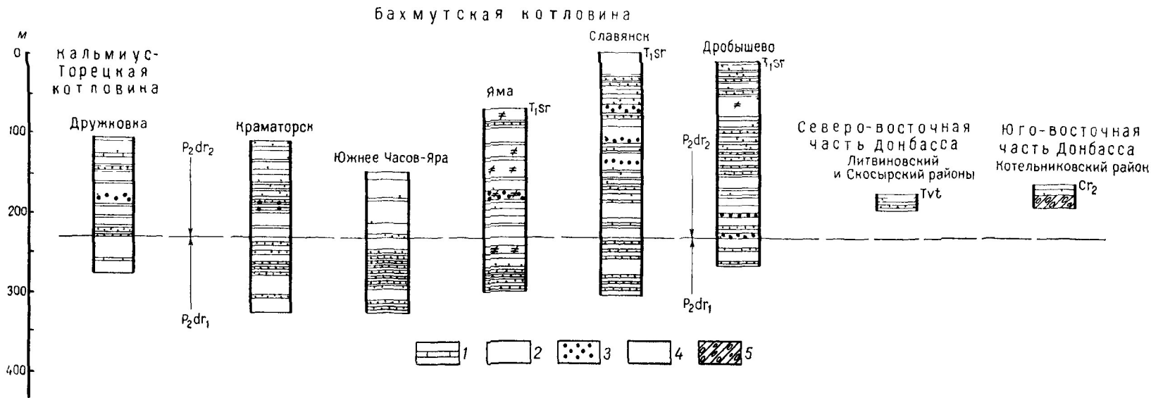
Рис 36 Сопоставление водоносных толщ дроновской свиты (по В.С. Кравченко литолого-стратиграфическое расчленение — по материалам треста «Артемгеология»)
