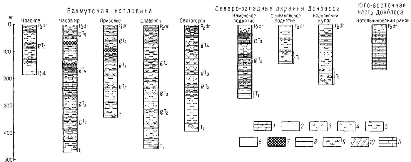
Рис. 35. Сопоставление водоносных горизонтов краматорской свиты (по В. С. Кравчѐнко, литолого-стратиграфическое расчленение — по материалам треста «Артемогеология», выделение свиты на Каменском и Сиваковском поднятиях — по Л П Нестеренко и М И Шамаеву)
