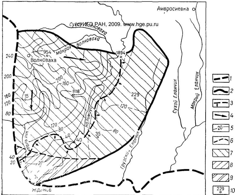
Рис 11. Карта распространения водоносного комплекса в кристаллических породах докембрия и продуктах их выветривания (Составила Н П Панкратьева)
