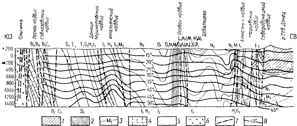
Рис 8. Схематический геотермический разрез Донецкого бассейна (По В. И. Свержевой и Е. А. Белецкой, 1963)
