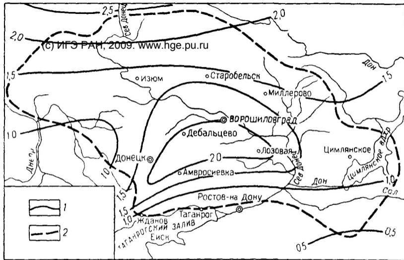
Рис 4. Среднегодовой сток с территории Большого Донбасса (л/сек·км 2 ) 1 — изолинии стока, 2 — граница Большого Донбасса
