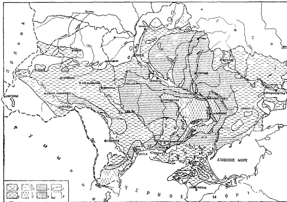
Рис 89 Карта просадочности лёссовых пород УССР. Составил В. Ф. Краев
