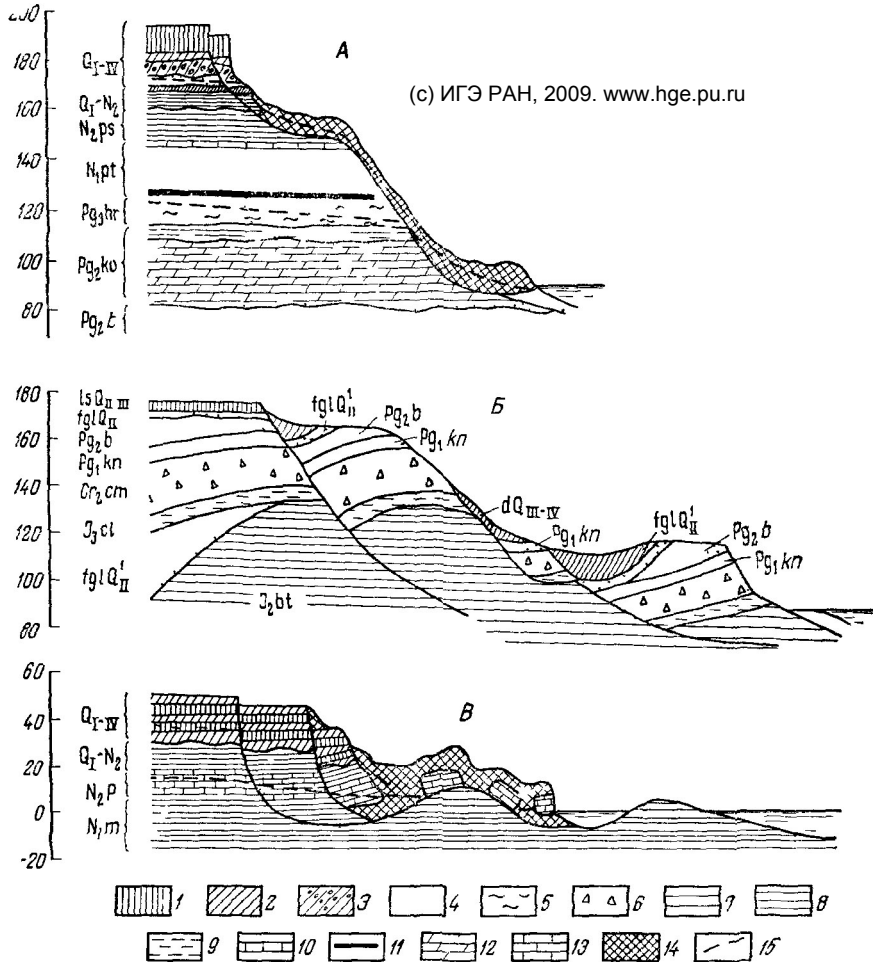
Рис 77 Схематические разрезы оползней
