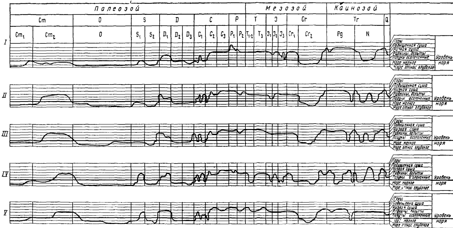
Рис. 43. Графики колебательных движений земной коры в пределах различных частей Вольно-Подольского артезианского бассейна I — наиболее погруженная часть (Львовская мульда); II — центральная часть; III — восточная краевая часть; IV — зона сопряжения платформы с Предкарпатским краевым прогибом; V — северная краевая часть
