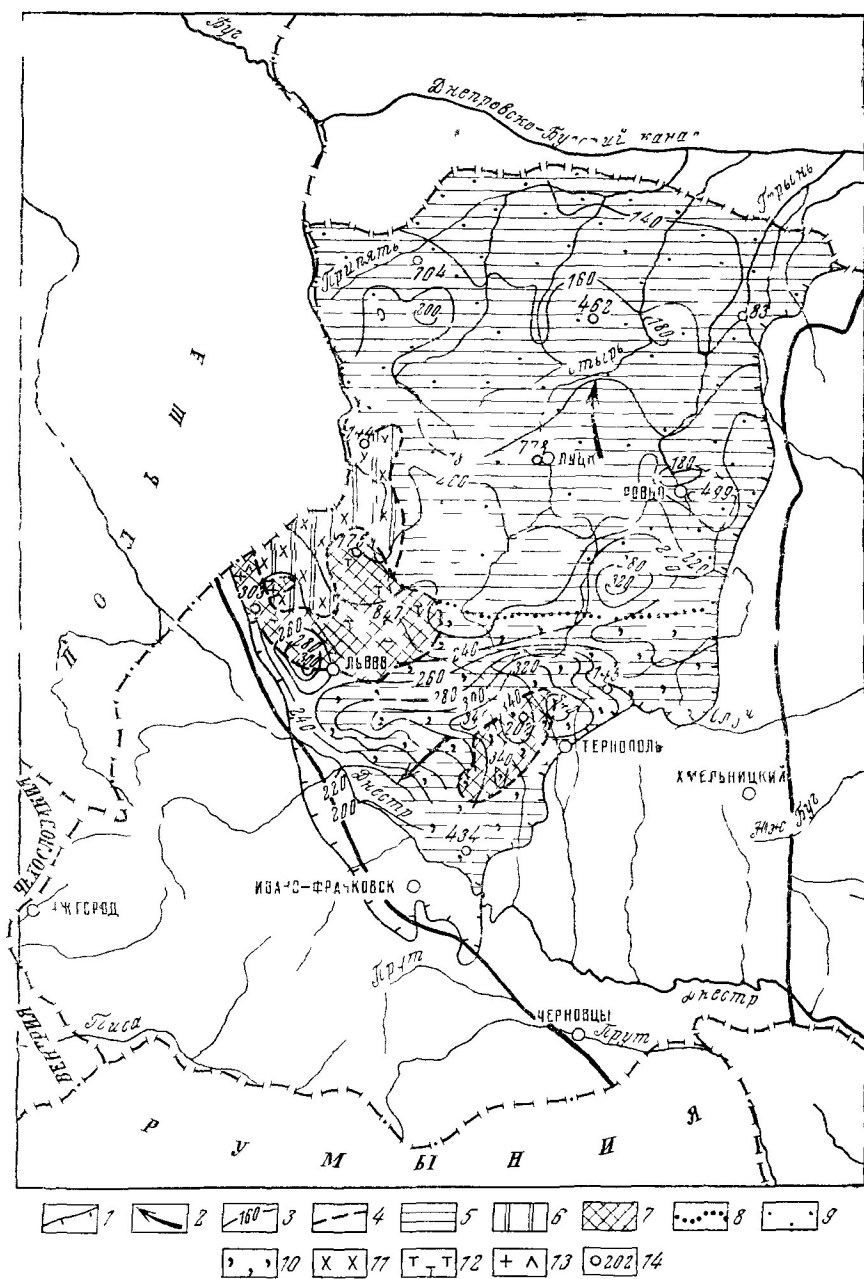
Рис 34 Карта распространения водоносного горизонта в мергельно-меловых отложениях сенон-турона Волино-Подольского артезианского бассейна (составили К Н Варава, Т С Николаенко)
