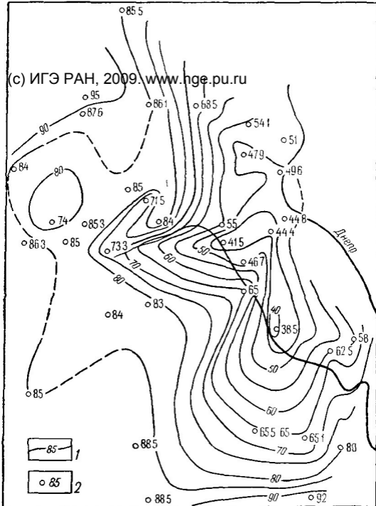
Рис. 27. Карта гидроизопьез водоносного горизонта в сеноман-келловейских отложениях (г. Киев, 1965 г.)
