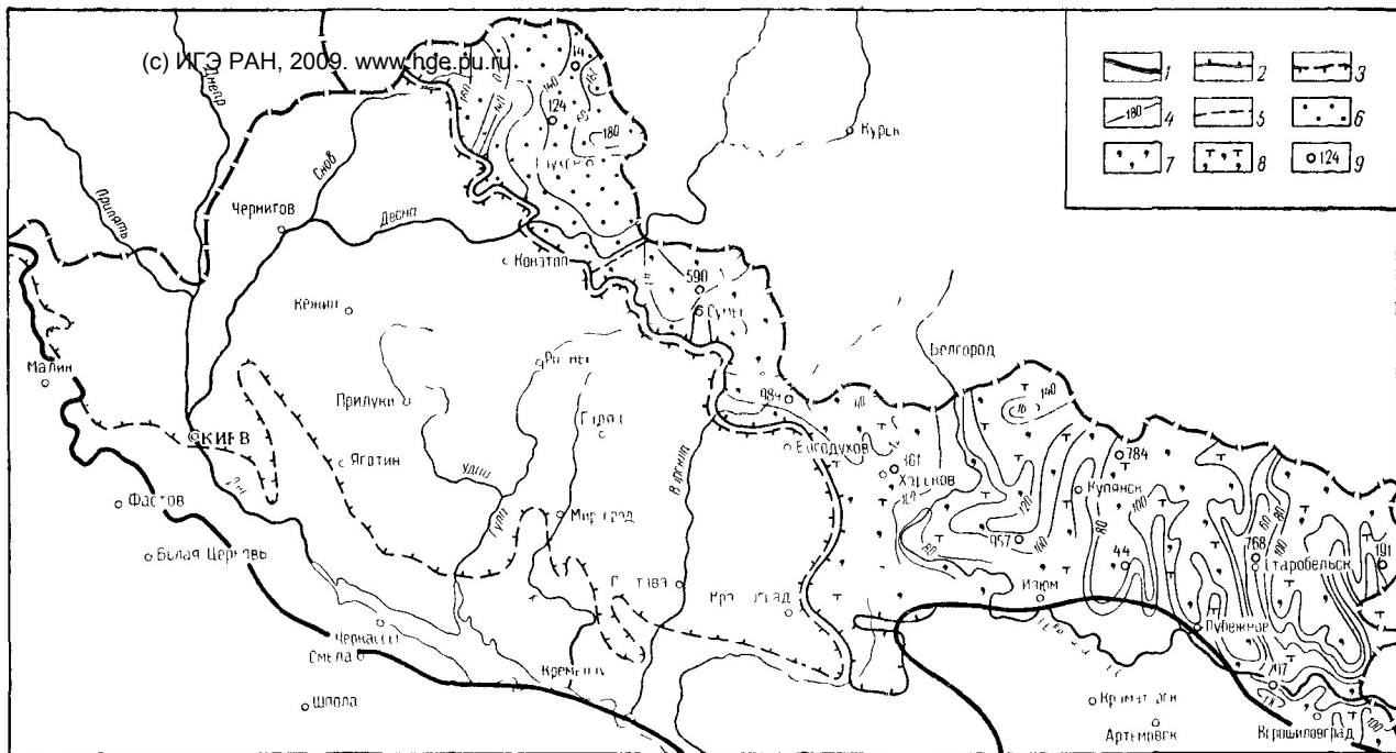
Рис 20. Карта распространения водоносного горизонта мергельно-меловых отложений Днепровско-Донецкого артезианского бассейна (составили Ю. Г. Головченко, Ж. С. Камзист)
