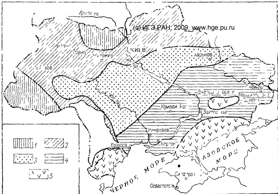
Рис. 8 Минерализация воды малых рек (по А. Д. Коиенко)
