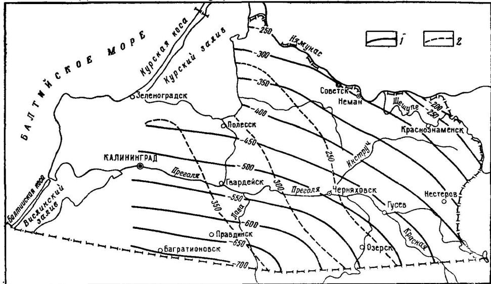
Рис. 8 Глубина залегания и мощность триасовых отложений
