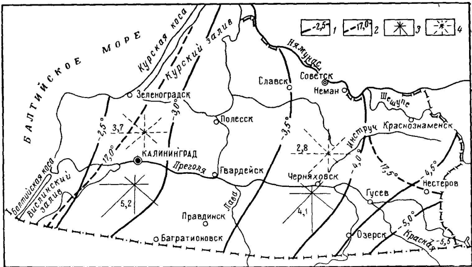
Рис 4. Температура воздуха, направление и скорость ветра в январе и в июле, по Ц Я. Дорфман, 1962
