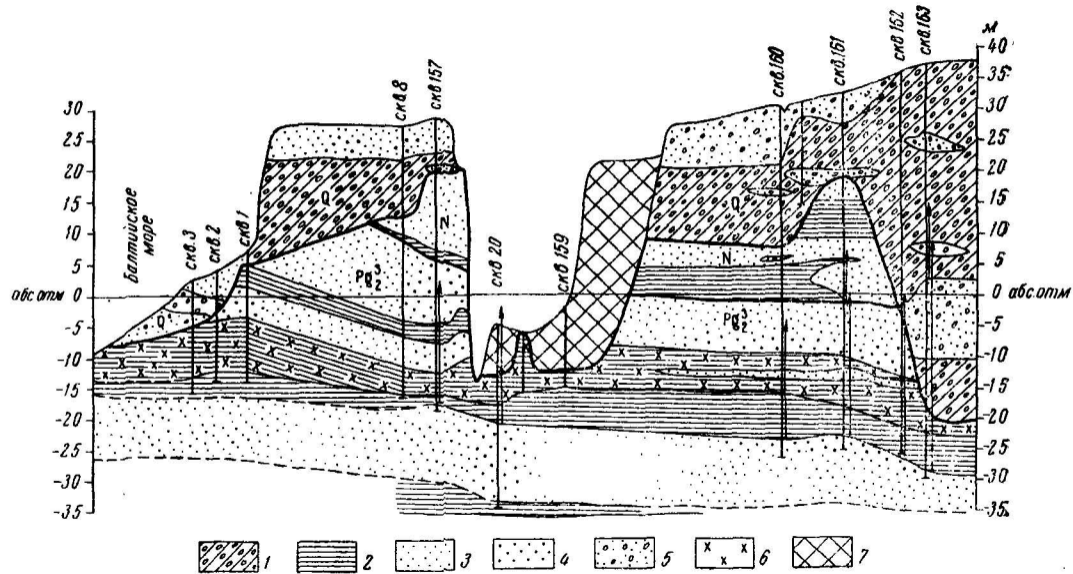
Рис. 24. Гидрогеологический разрез месторождения «Янтарное»
