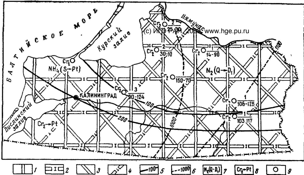
Рис. 23. Схема распространения минеральных вод
