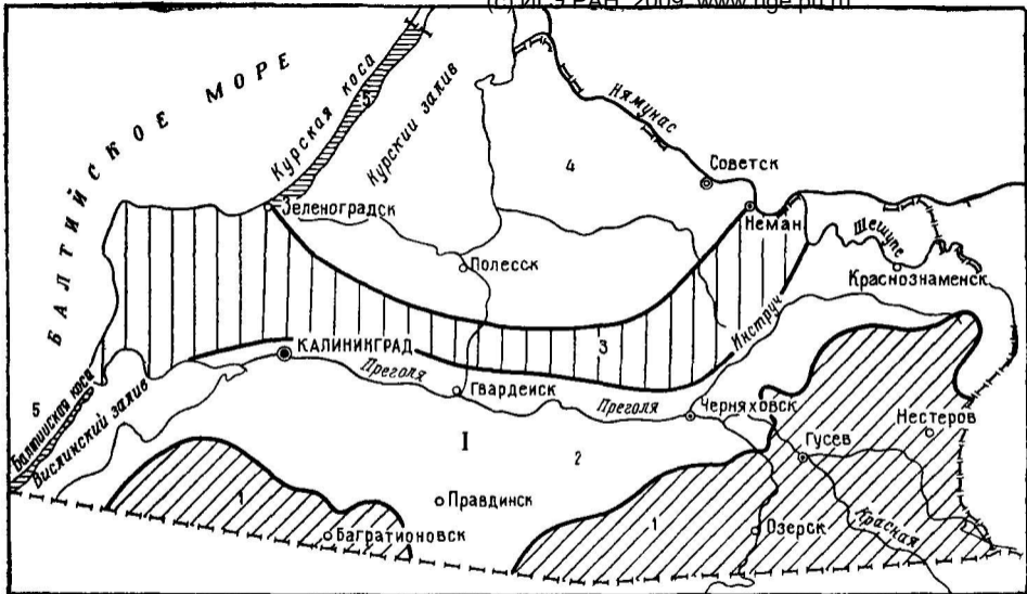
Рис 21 Карта гидрогеологического районирования
