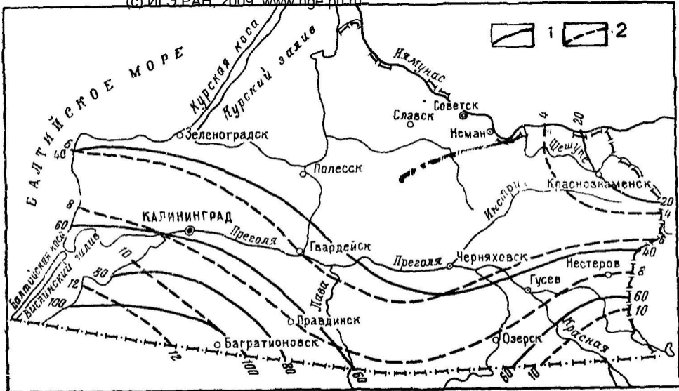
Рис. 18. Схема распределения слоя и коэффициентов подземного стока, по И. А. Игнатовичене и А. Р. Кондратасу
