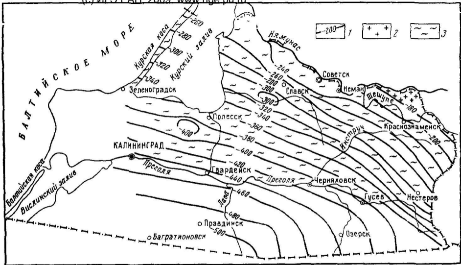
Рис. 14. Гидрогеологическая схема нижнеюрско-среднекеellowейского водоносного горизонта 1 — стратонизогипсы кровли в м абс.; 2 — воды сильносоленоватые (3—10 г/л), 3 — воды слабосоленоватые (10—25 г/л)
