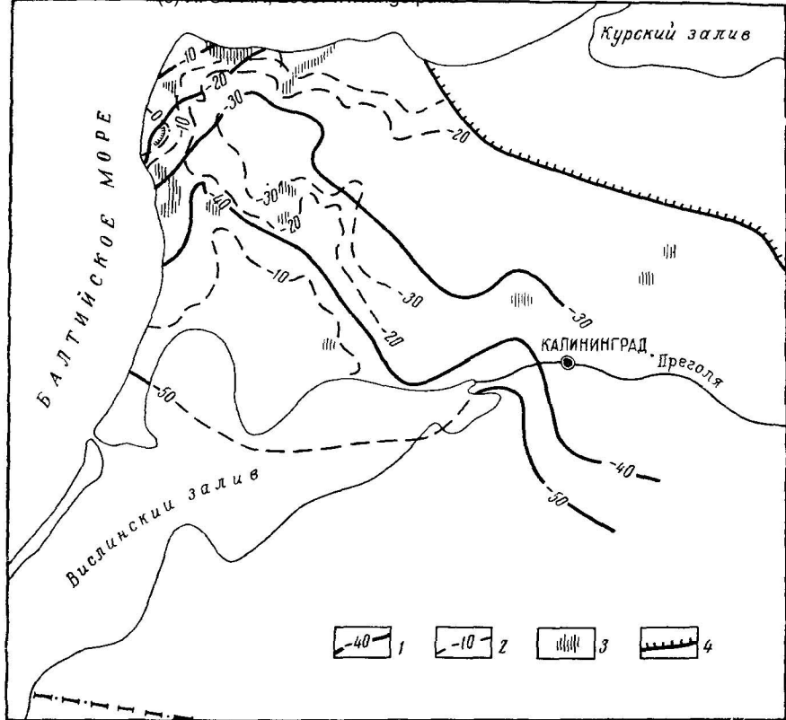
Рис 12. Гидрогеологическая схема палеогенового водоносного горизонта (нижнего) 1 — стратизогипсы кровли в м, 2 — пьезозогипсы в м, 3 — места отсутствия водоносного горизонта, 4 — граница распространения водоносного горизонта
