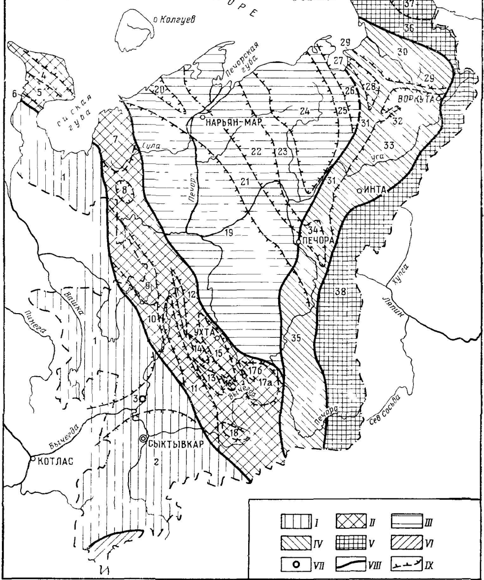
Рис 9. Схема тектонического строения территории Коми АССР и Ненецкого национального округа (составил К К Воллосович)
