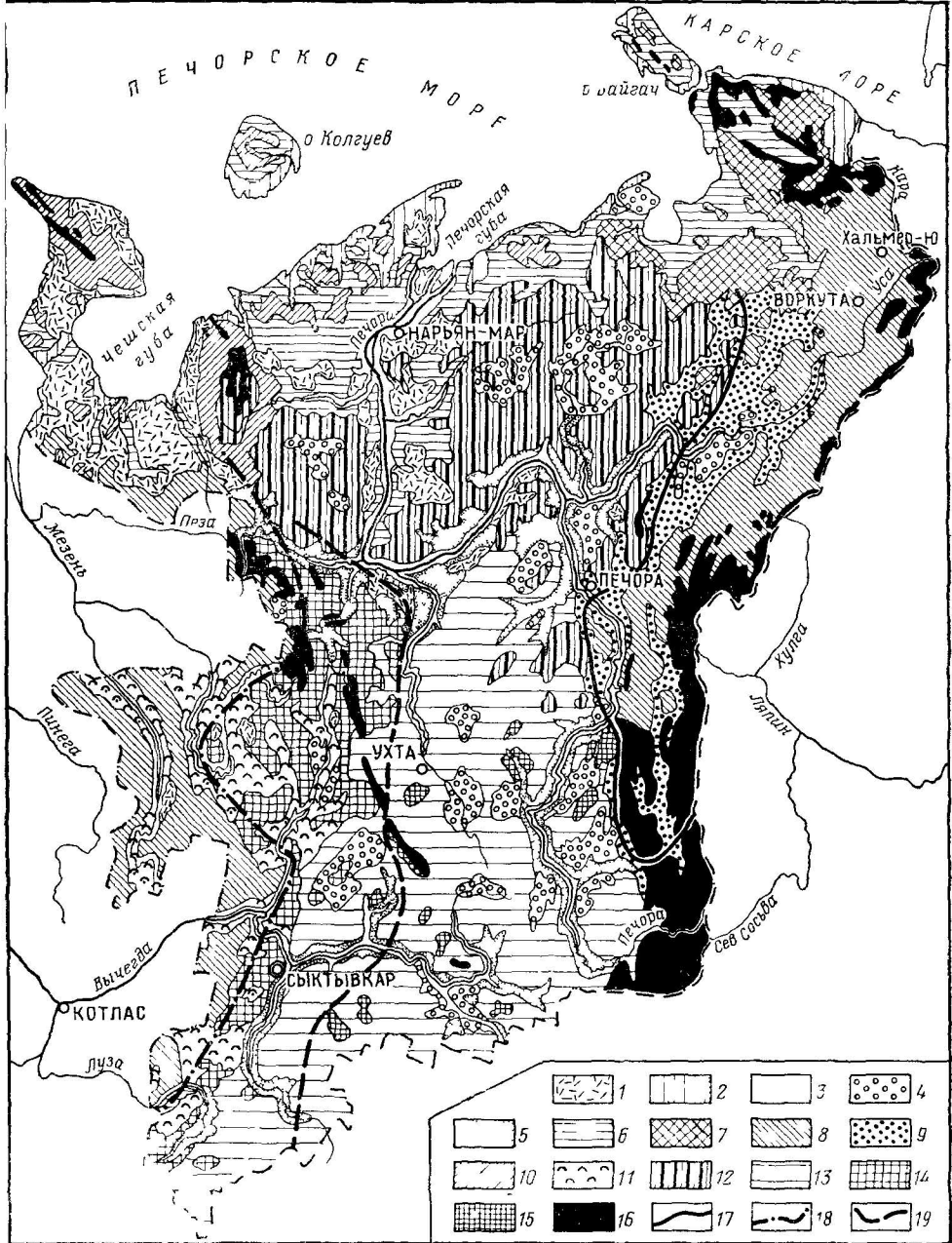
Рис 8 Карта четвертичных отложений Коми АССР и Ненецкого национального округа (составили К. К. Воллосович и С. И. Закревский, 1965 г.)
