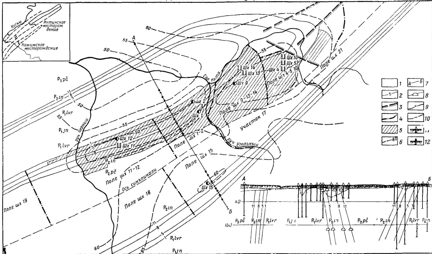
Рис. 28. Схематическая гидрогеологическая карта Интинского месторождения (составили И. А. Конжин и Н. Б. Какунов)
