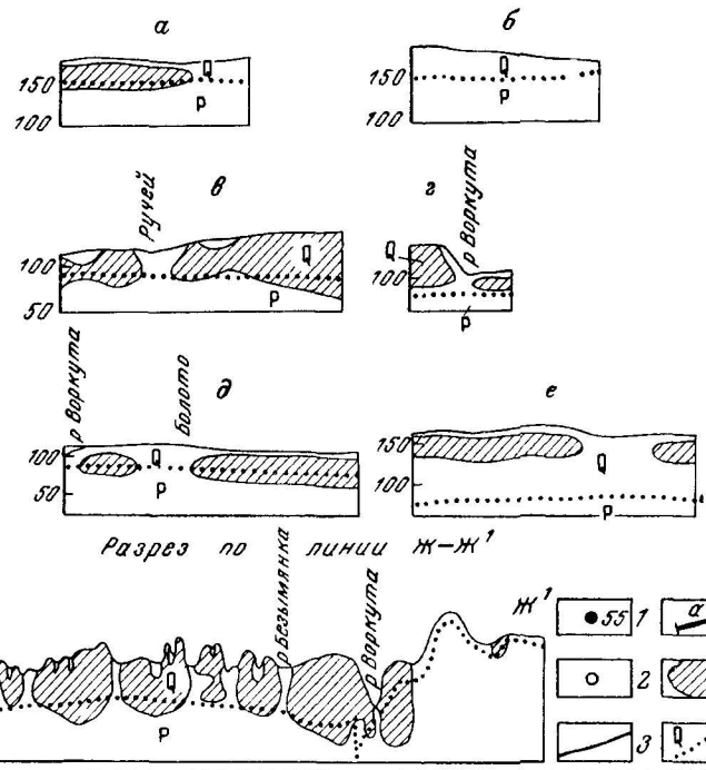
Рис 23 Характеристика мощностей мерзлых пород на Воркутском месторождении (составил Н. Б. Какунов) 1 — установленная мощность мерзлых пород по скважине, 2 — скважина, пройденная в талике, 3 — контур месторождения 4 — линия разреза На разрезах 5 — мерзлые породы, 6 — контакт четвертичных и пермских пород а-б-в-г-д-е — детали строения мерзлых пород
