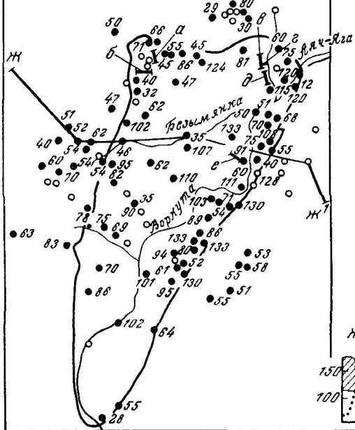
Рис 23 Характеристика мощностей мерзлых пород на Воркутском месторождении (составил Н. Б. Какунов) 1 — установленная мощность мерзлых пород по скважине, 2 — скважина, пройденная в талике, 3 — контур месторождения 4 — линия разреза На разрезах 5 — мерзлые породы, 6 — контакт четвертичных и пермских пород а-б-в-г-д-е — детали строения мерзлых пород
