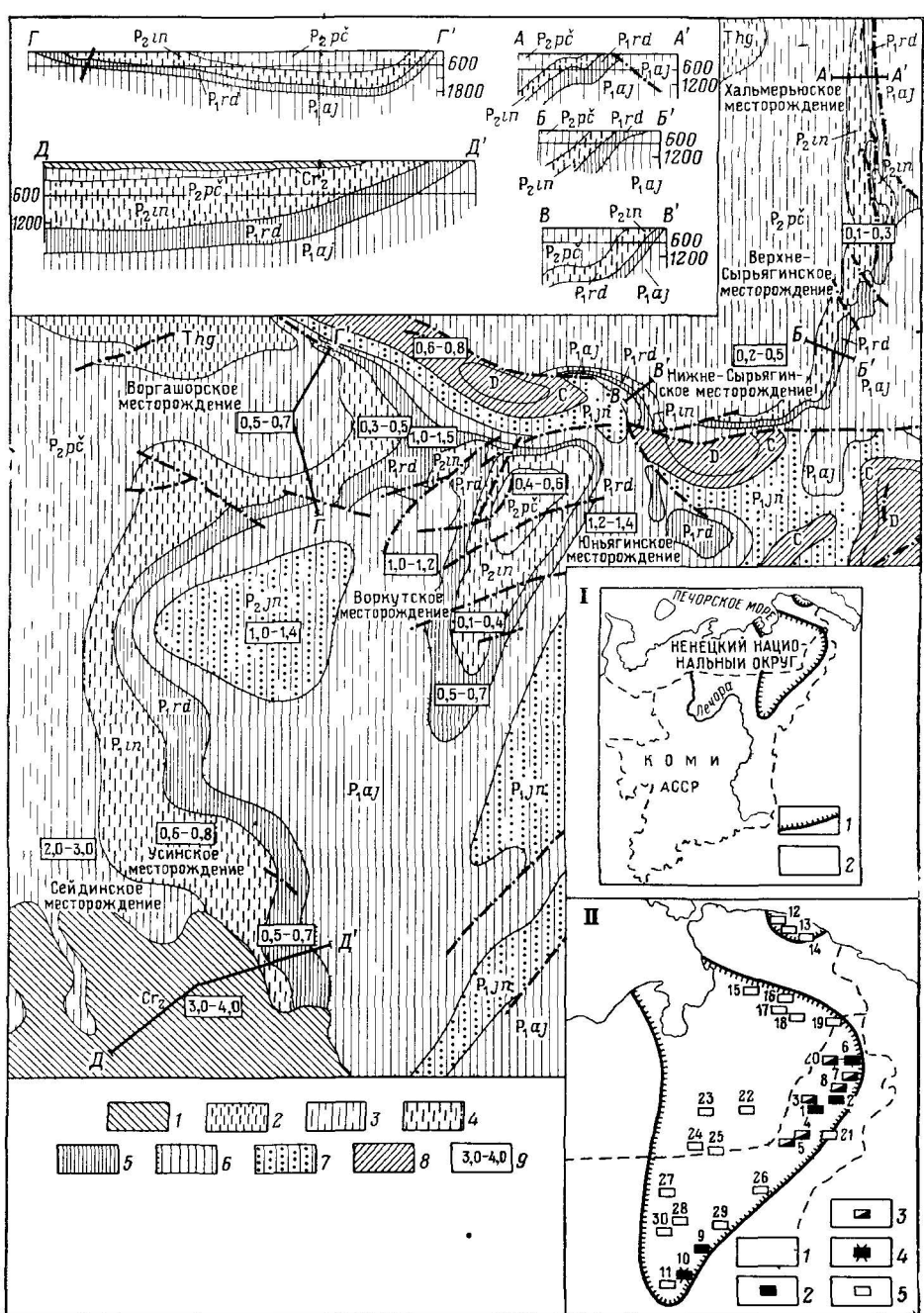
Рис 21 Схематическая гидрогеологическая карта северо-восточной части Печорского угольного бассейна с обзорными схемами (врезками I и II) расположения угольных месторождений (составил Н. Б. Какунов)
