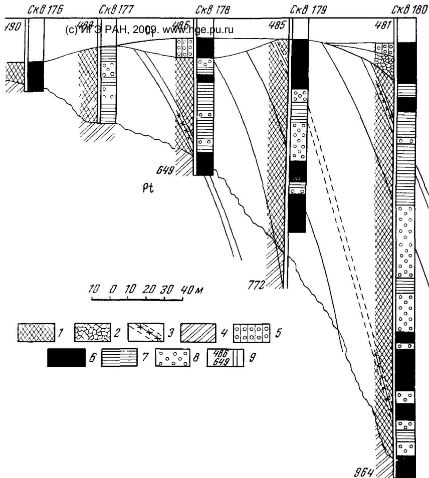
Рис 100. Инженерно геологический разрез рудной залежи Яковлевского месторождения (по материалам ГУЦР)
