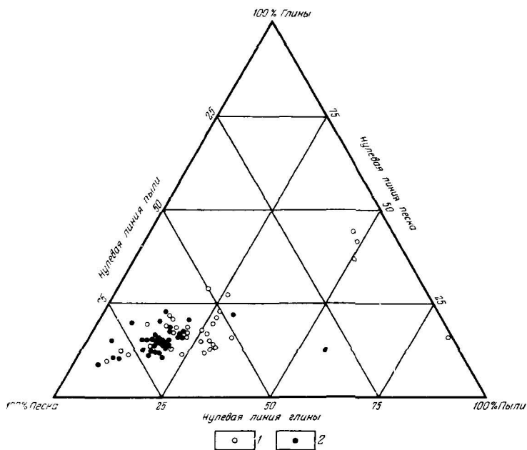
Рис 96 График гранулометрического состава юрских отложений Лебединского месторождения По Г Г Скворцову и Л И. Романовской
