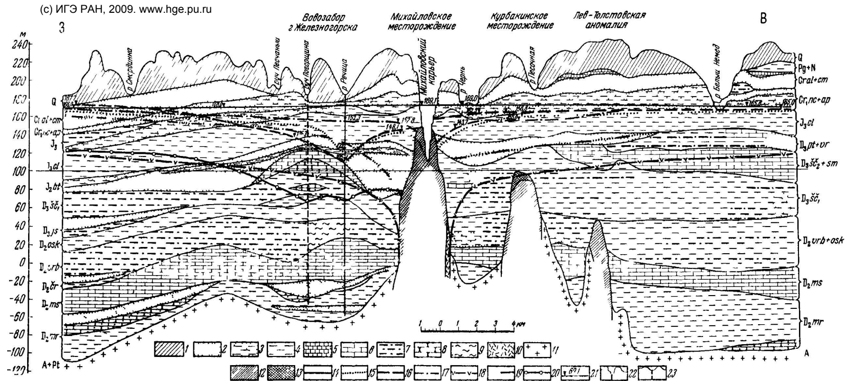
Рис 66 Гидрогеологический разрез по Михайловскому железорудному району (вкрест простирания рудных залежей) Составил В С Плотников и др.
