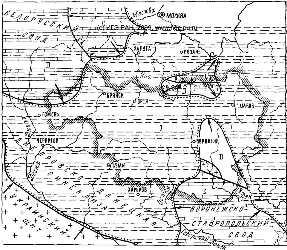
Рис 42 Схематическая палеогидрогеологическая карта ранней и средней юры Составила Г Н Плотникова Условные обозначения см к рис 39
