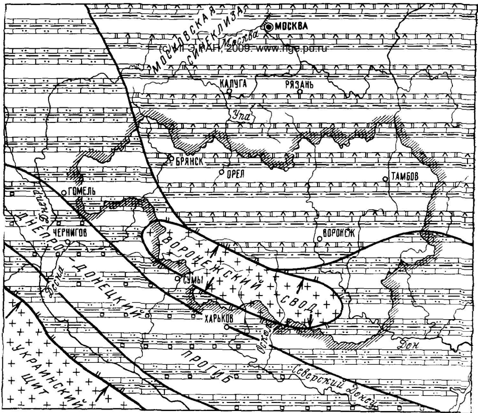
Рис. 40. Схематическая палеогидрогеологическая карта среднего девона — турне. Составила Г. Н. Плотникова. Условные обозначения см. к рис. 39
