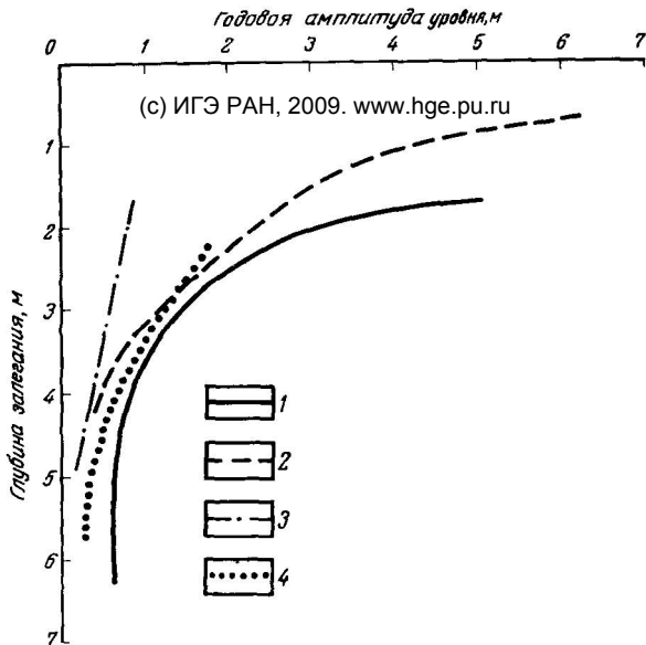
Рис. 21. График зависимости амплитуды колебания уровня грунтовых вод от средней годовой глубины залегания уровня Составил В А Коробейников
