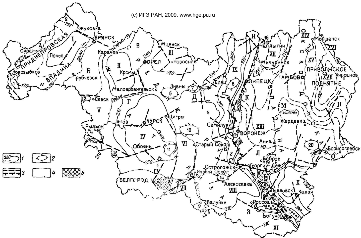
Рис. 13. Схема неотектонических структур Составил Г. И. Раскатов
