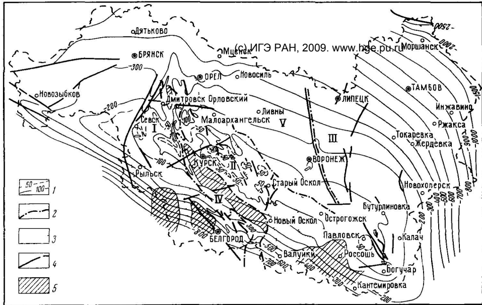
Рис 11 Схема тектоники и современного рельефа докембрия Воронежской антеклизы. Составил Д. Н. Утехин
